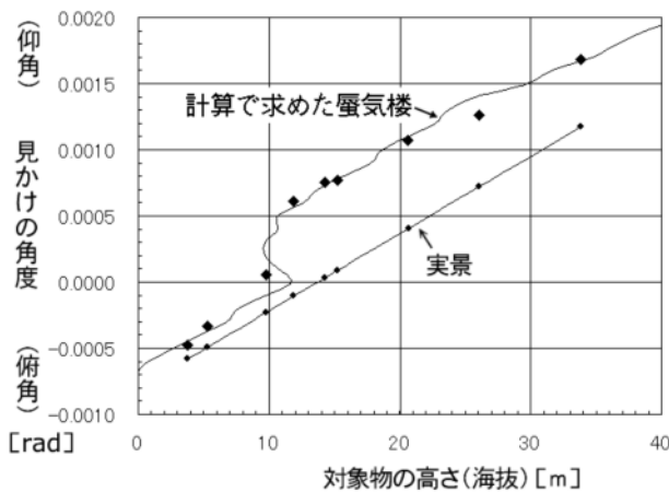
図6 求めた屈折率による蜃気楼の変形プロファイル
