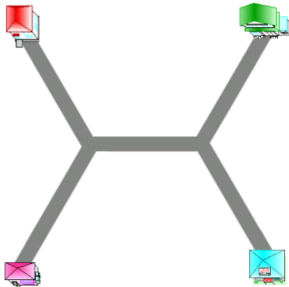
図4 4軒の家を結ぶ最短経路
