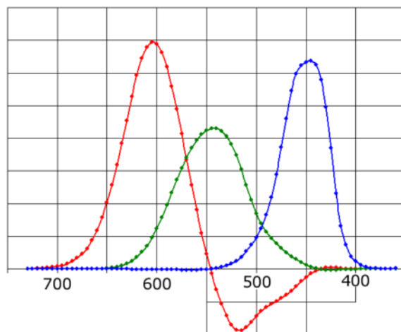
図1 光の三原色で表わせない色が存在することを示すグラフ
